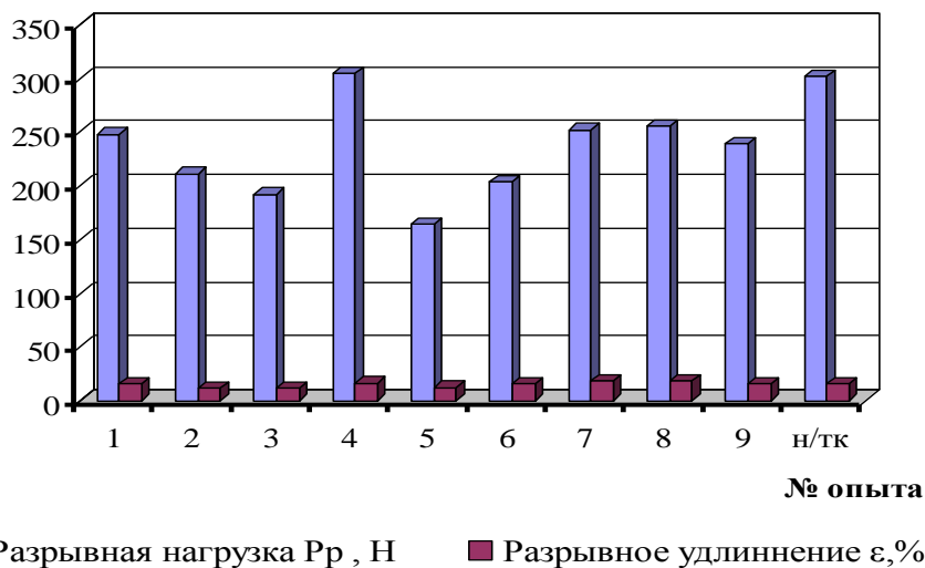
Рисунок 1 – Показатели прочности хлопчатобумажной ткани (I группа) в зависимости от концентрации компонентов композиции (по основе)
