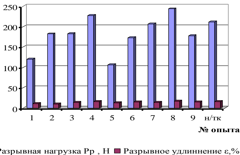
Рисунок 2 – Показатели прочности хлопчатобумажной ткани (I группа) в зависимости от концентрации компонентов композиции (по утку)
