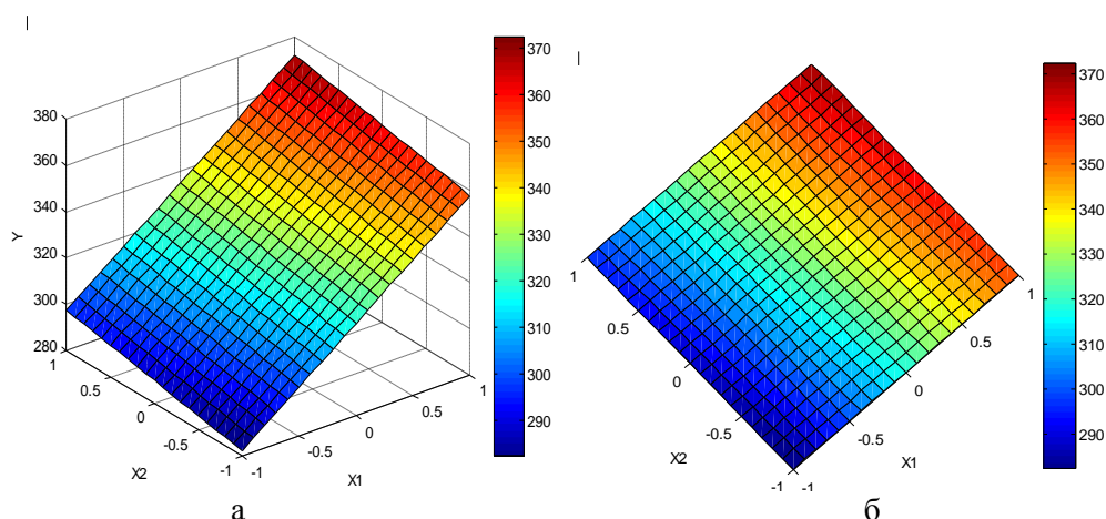
Рисунок 1 – Изменение разрывной нагрузки (Н) обработанной ткани в зависимости от концентраций СК ( x_1 ) и \text{CuSO}_4 ( x_2 ): а – трехмерный график; б – двухмерный график
