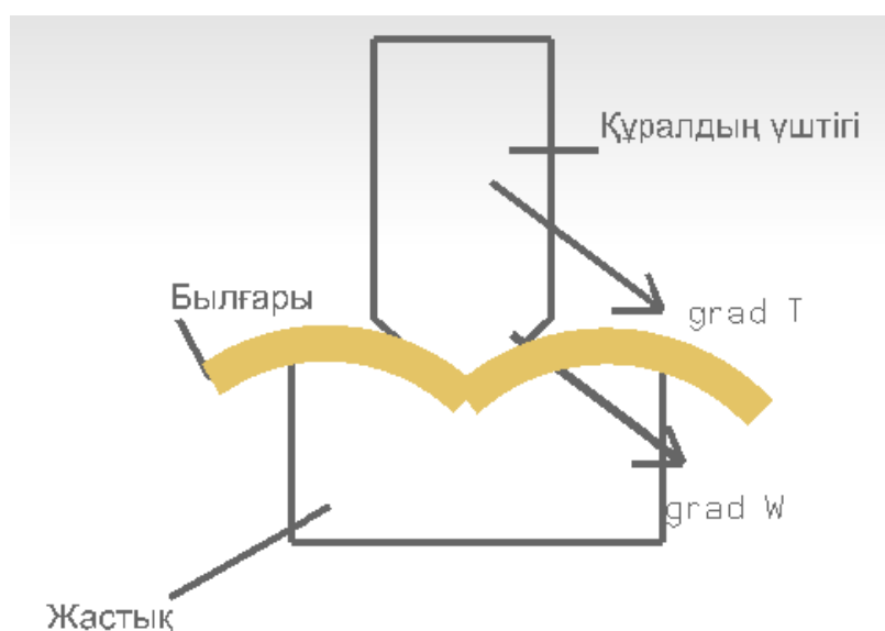
Сурет 3 – Дайындаманы жанастырып қыздырудағы жылу алмасуы
