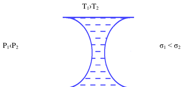
Сурет 2 – Капиллярлы қопсы дененің термоылғалөтімдік схемасы (мұндағы: температура, беттік қысым, беттік кернеу)
